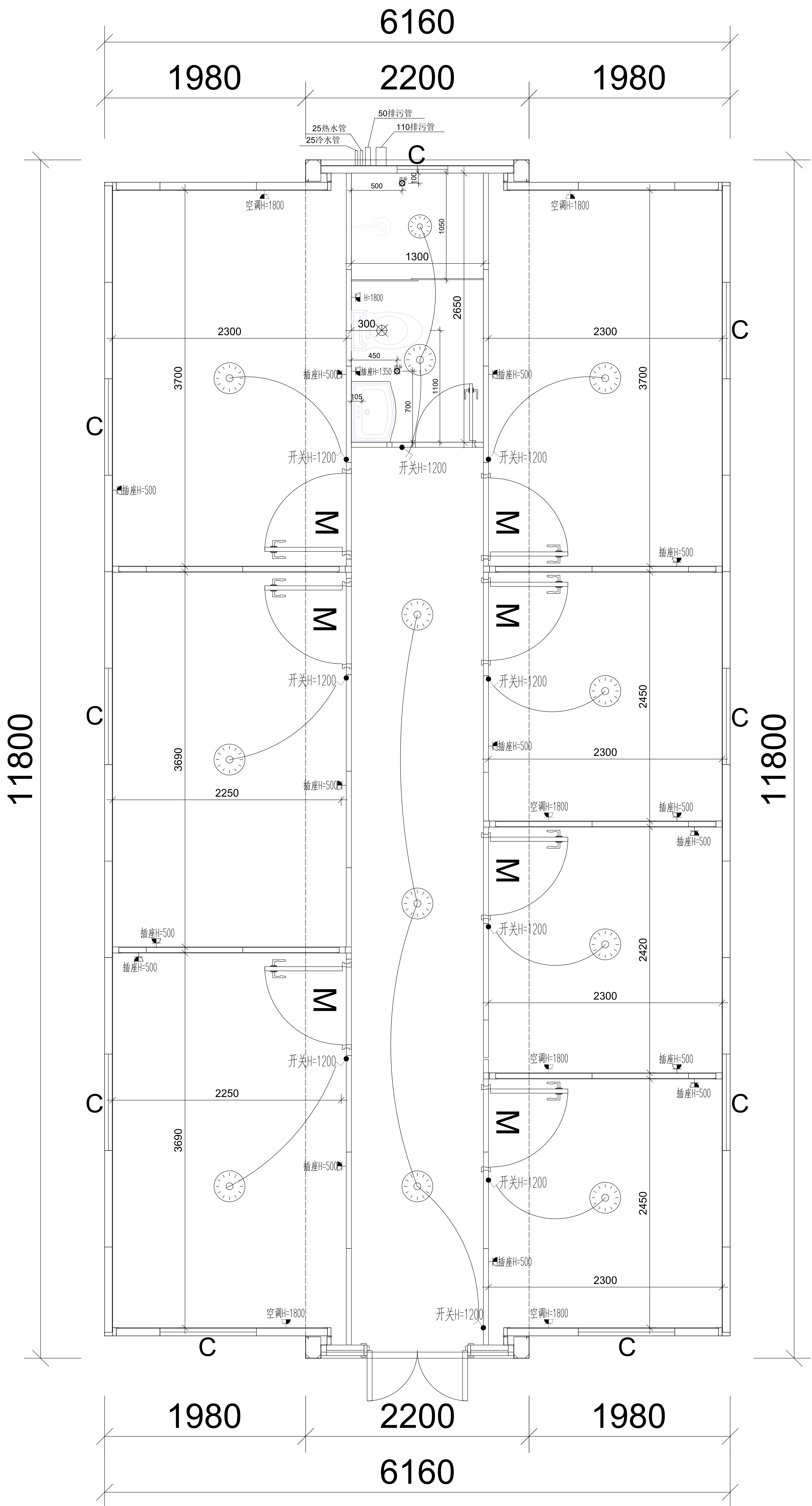
40尺7室卫平面图
