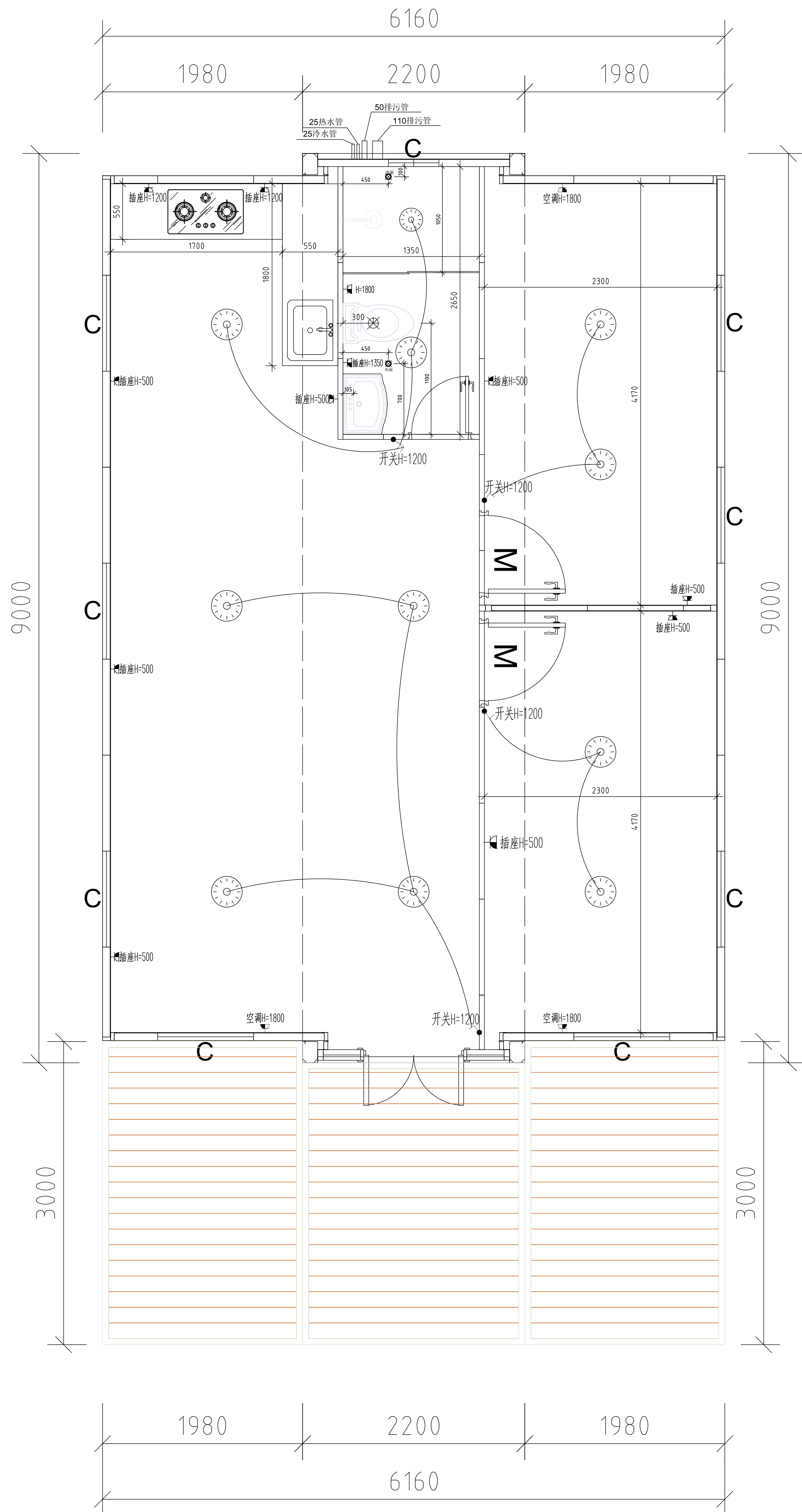
30尺2室1厅1厨1卫平面图
