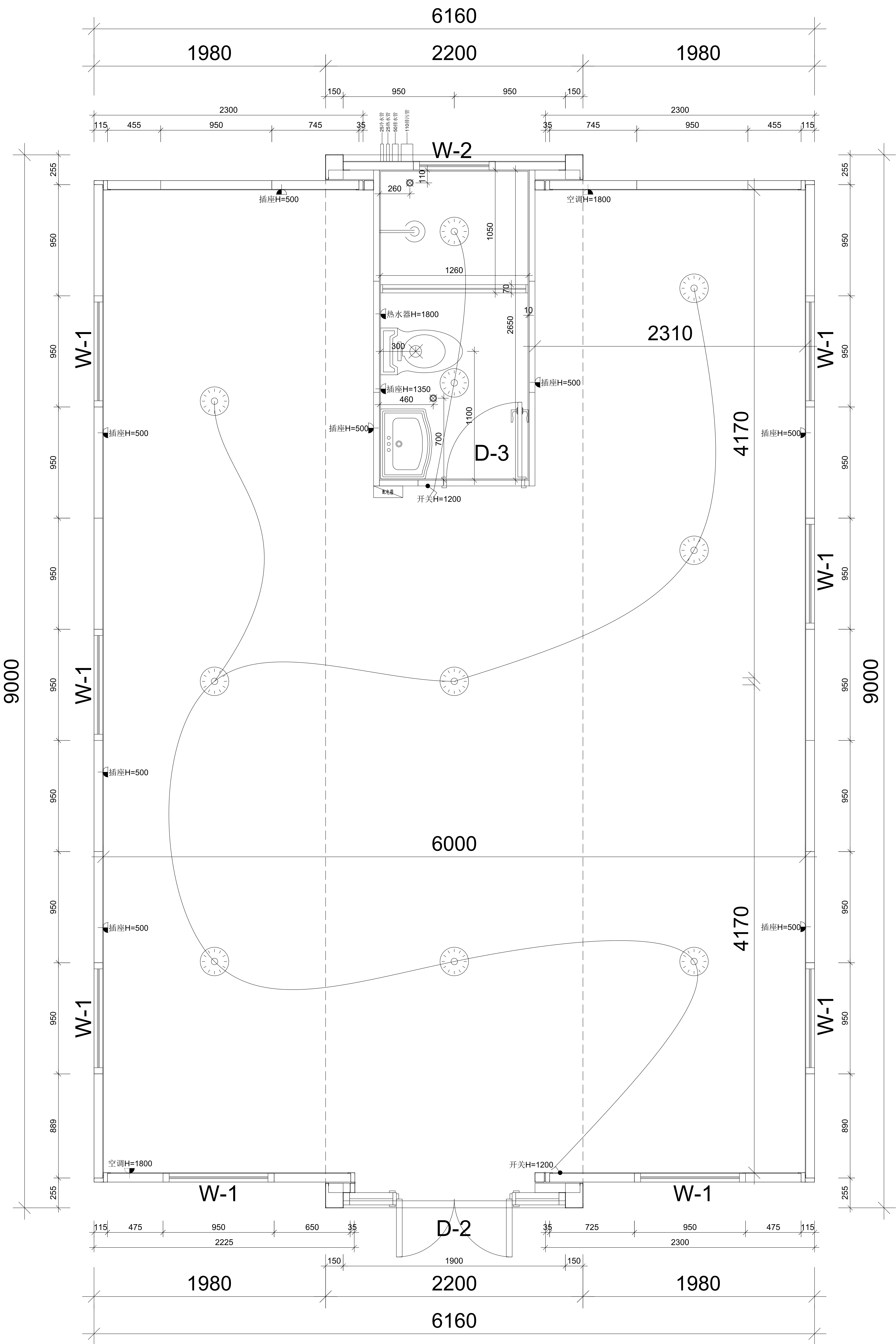
30尺1厅1卫平面图
