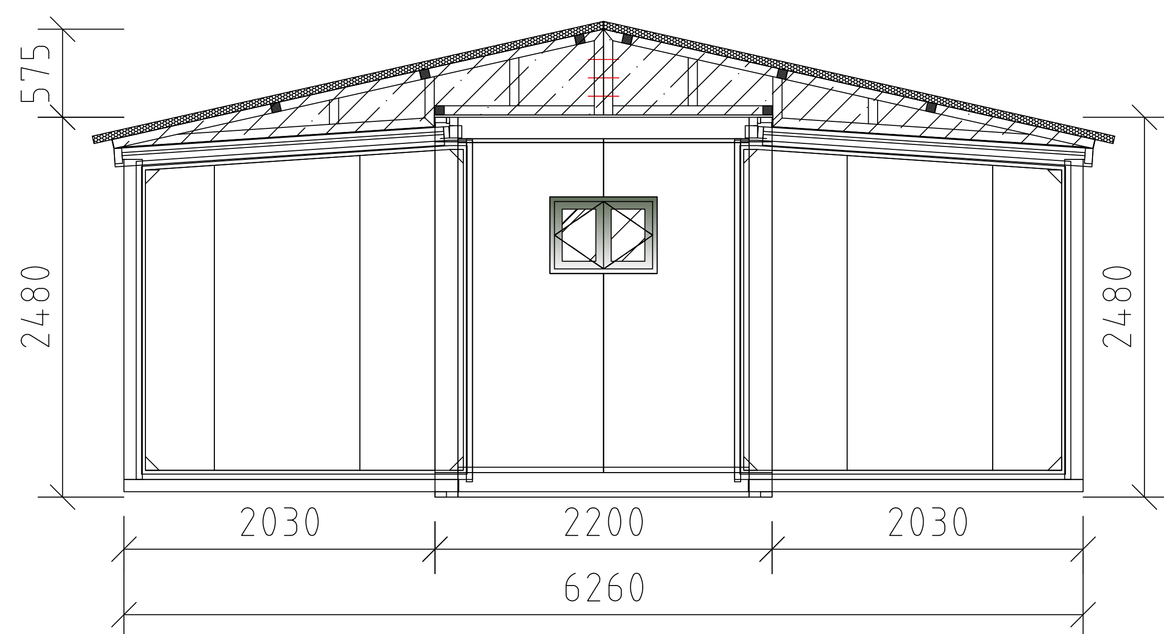
20尺北立面图
