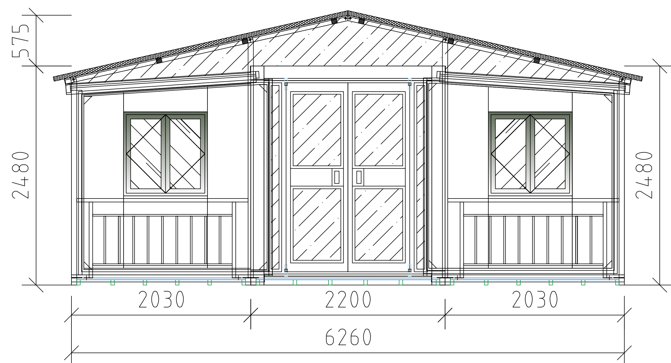
20尺南立面图
