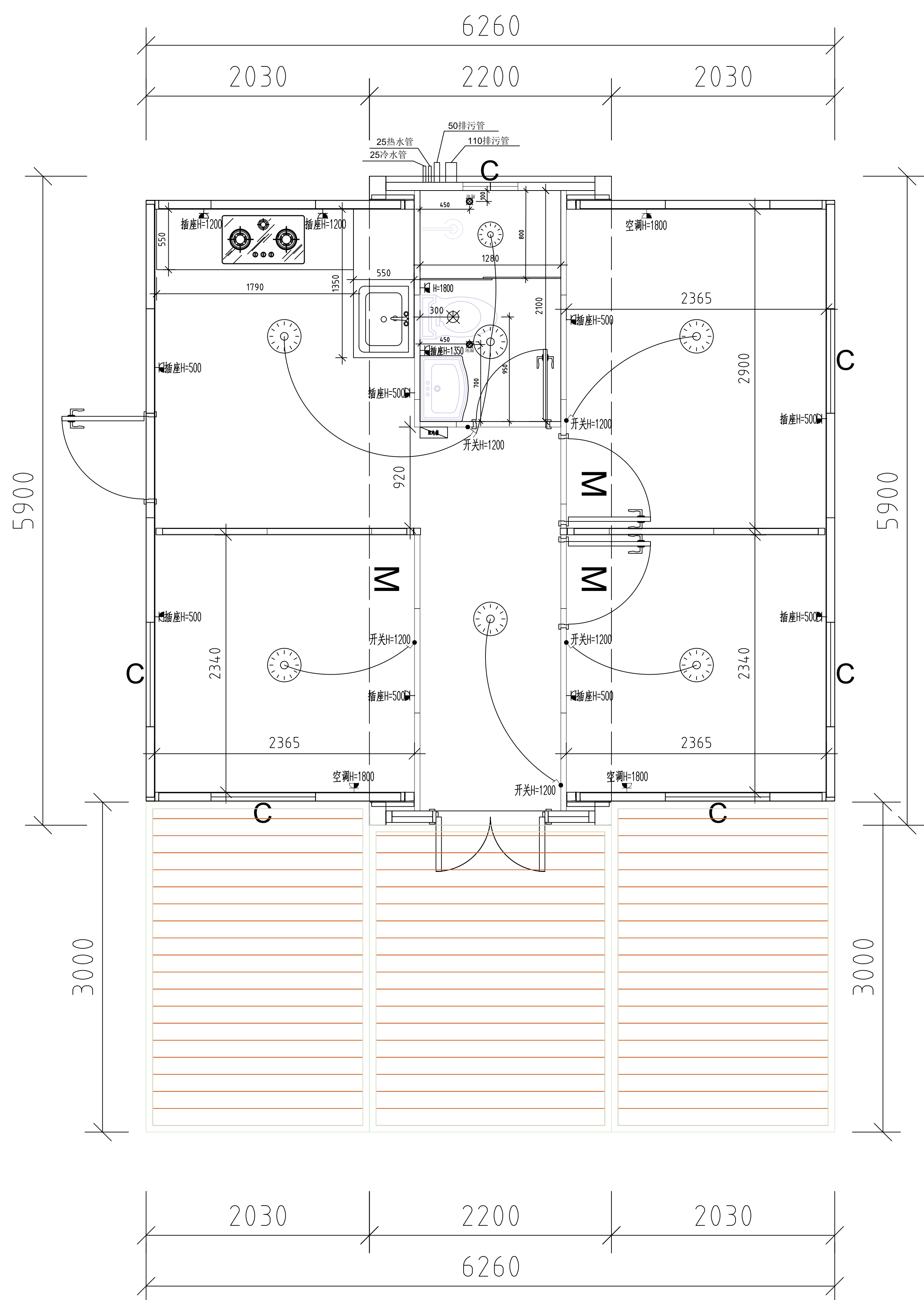
20尺3室1厨1卫平面图
