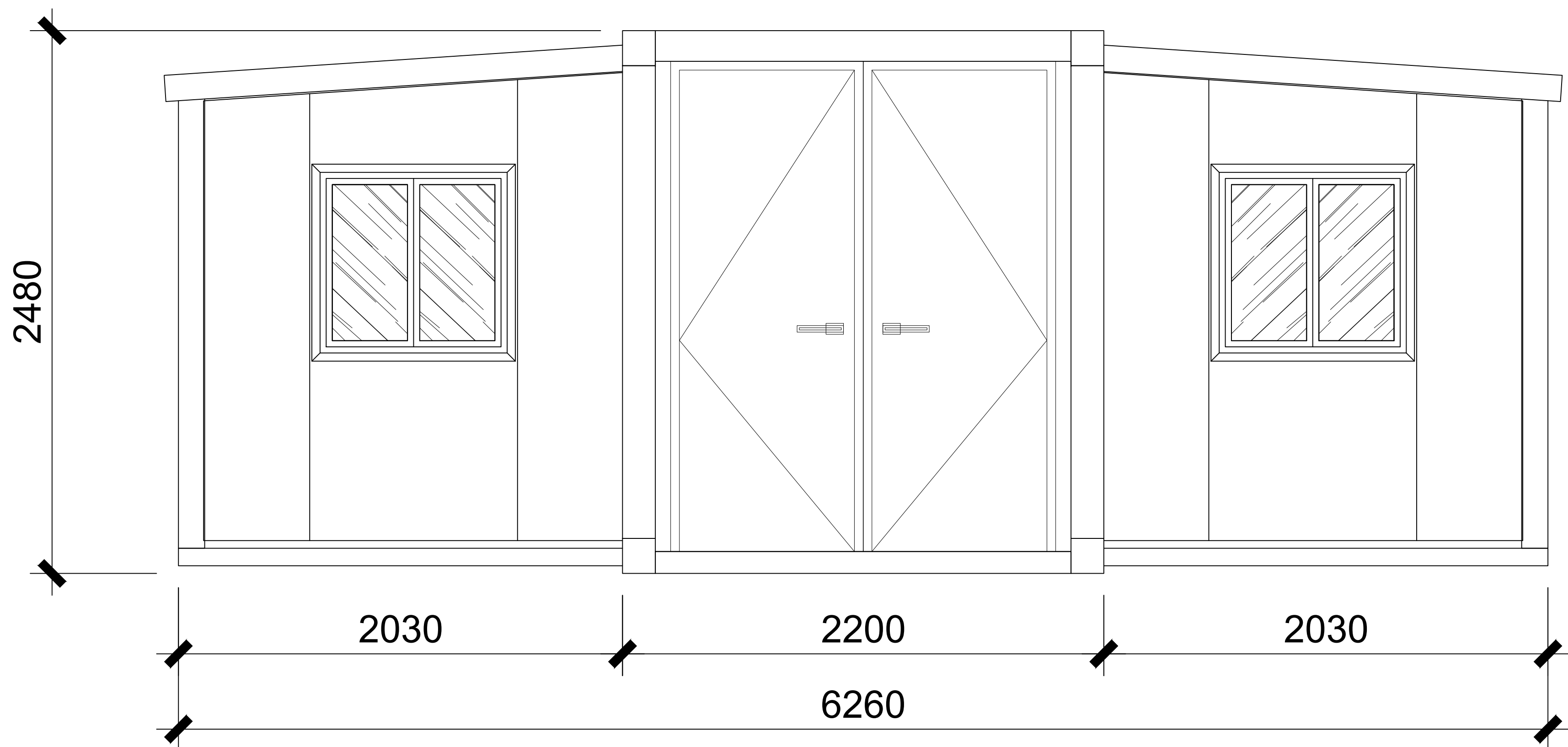
前立面
