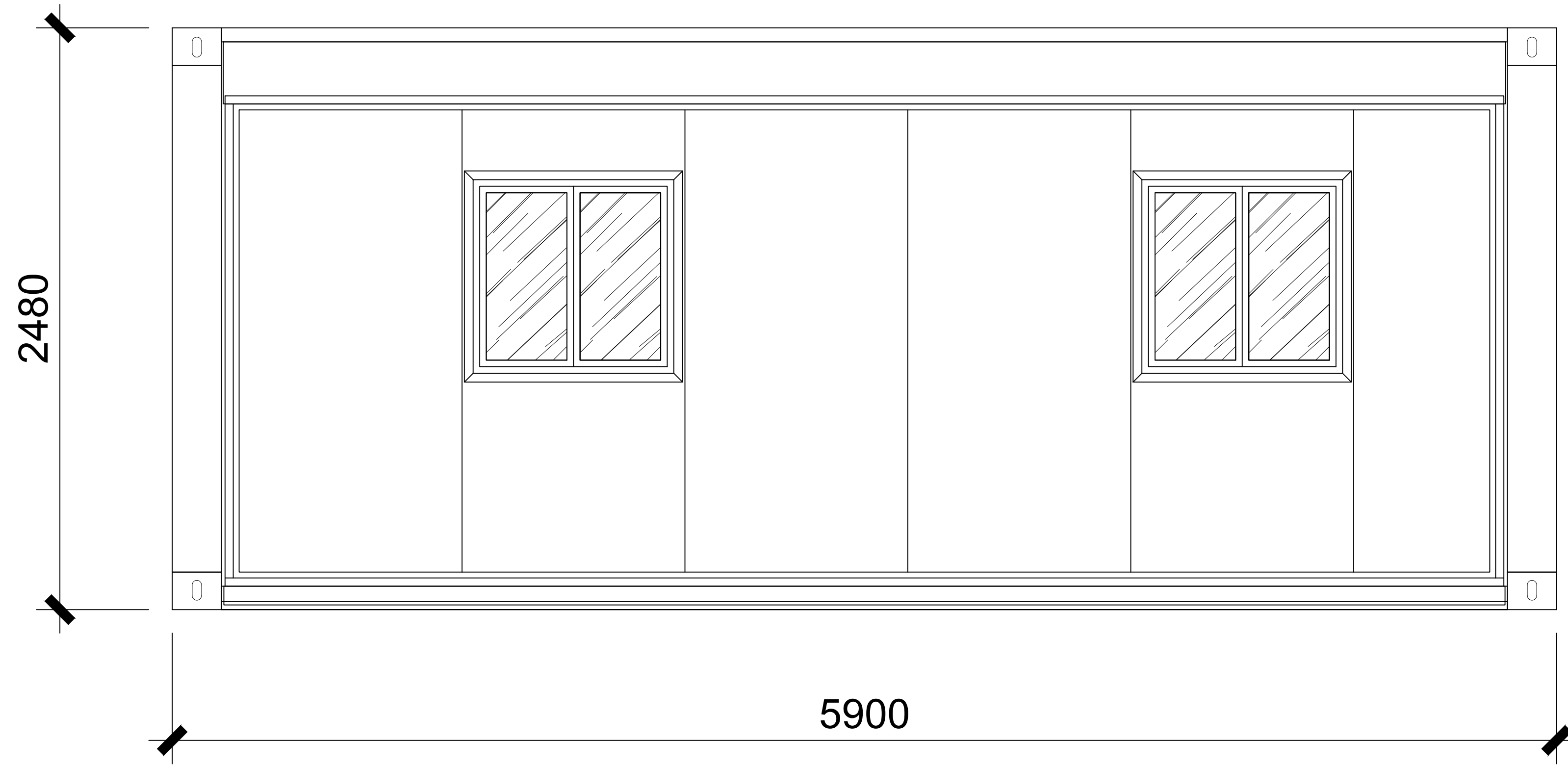
右立面
