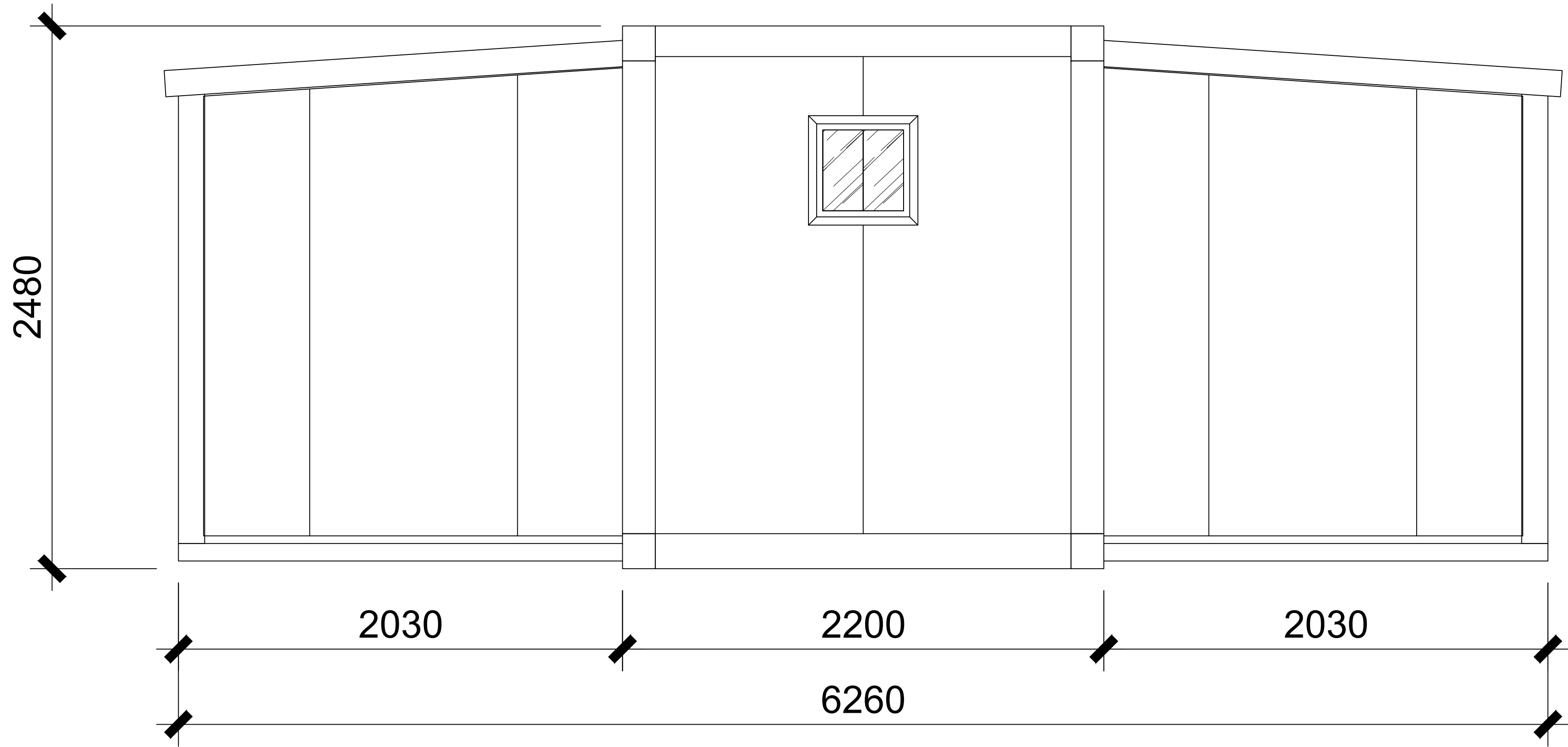
后立面
